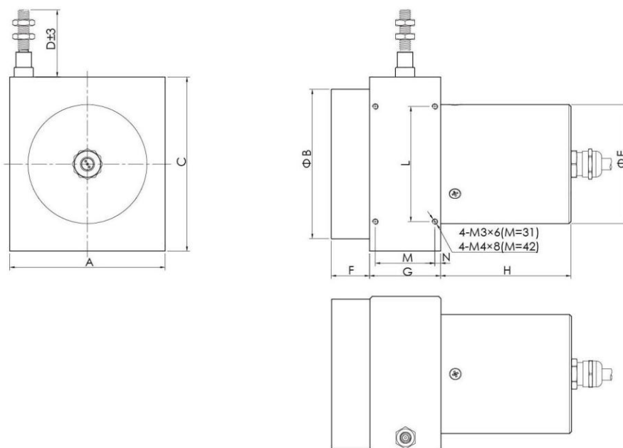
外形尺寸图 Dimensions
